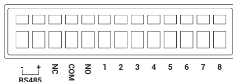
Рис. 2.1 Интерфейс подключения (данные о порте энергопровода содержатся в указаниях на заводской табличке с паспортными данными)
