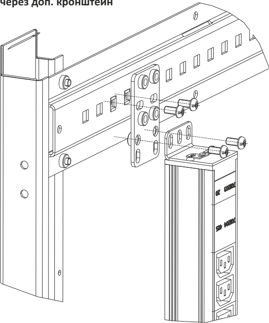
Схема 1 Крепление в шкаф ШТК-С-45U через доп. кронштейн
