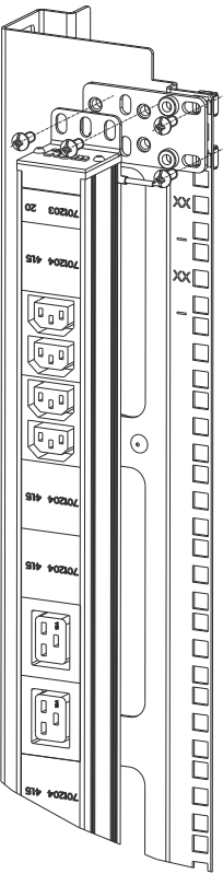
Схема 3 Крепление в шкаф ШТК-С-47U через доп. кронштейн
