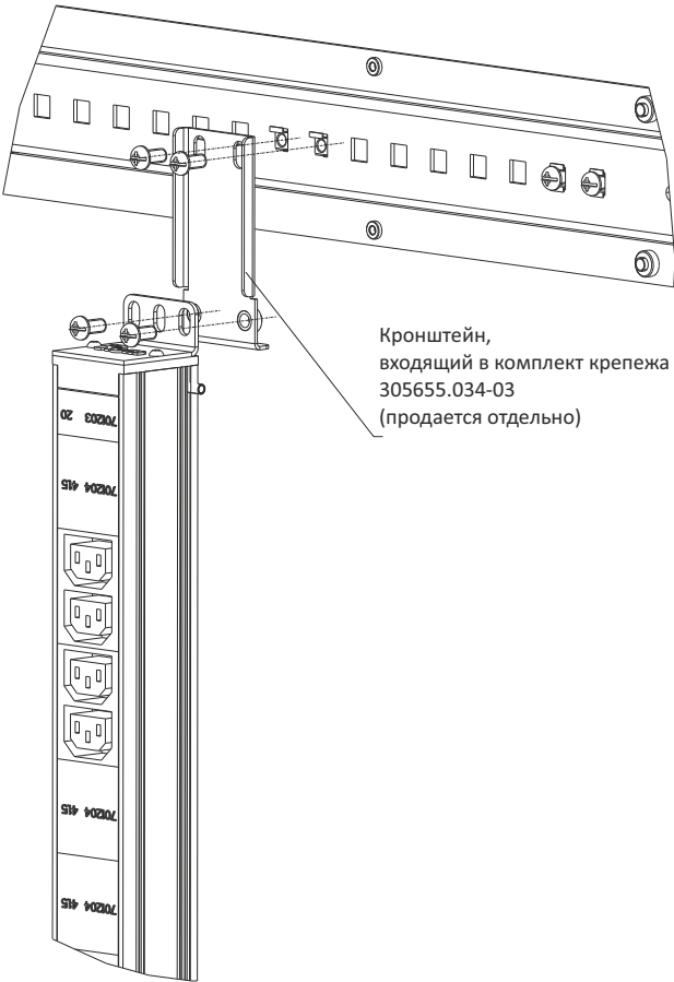
Схема 4 Крепление вертикального БР на юнитовую направляющую ШТК-СП через доп. кронштейн
