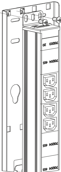
Схема 4 Крепление вертикального БР на юнитовую направляющую ШТК-СП через доп. кронштейн
