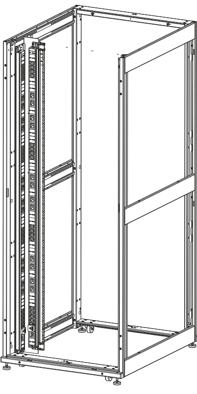
Установка БР в ШТК-СП 42-8-10
