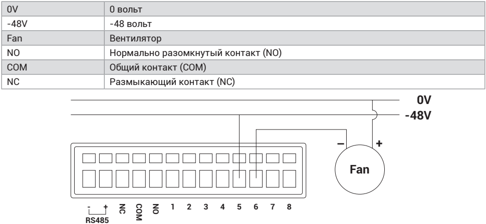
Рис. 2.3 Схема подключения интерфейса входа постоянного тока
