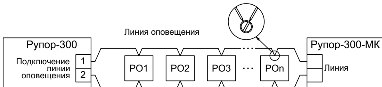
Рисунок 2. Подключение модуля Рупор-300-МК.
