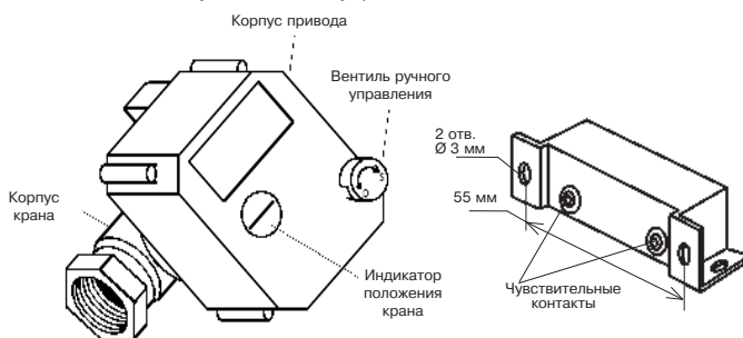
Рисунок 2 - Кран
