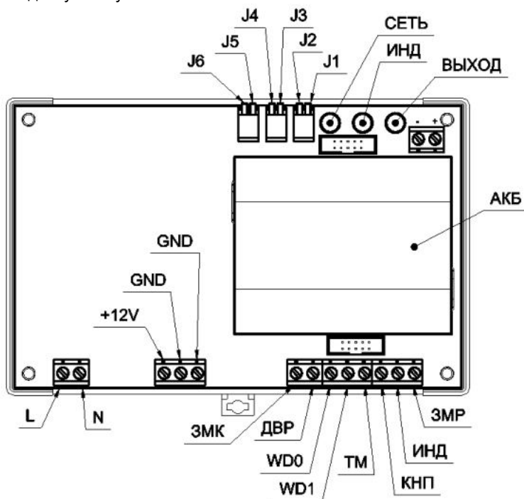
Рисунок 1 – Элементы подключения.
