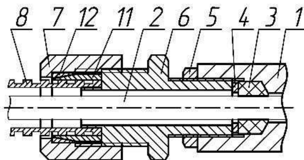
KB-15, KB-18, KB-20, для монтажа кабелем в металлорукаве
