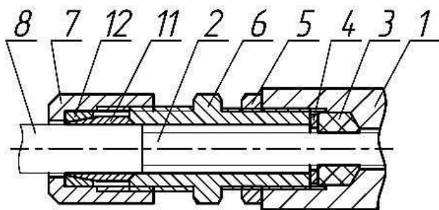
KB-12, для монтажа кабелем в металлорукаве или бронированным кабелем
