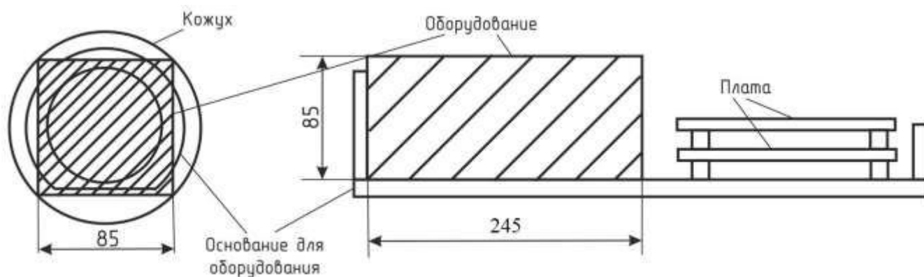
Рисунок 2 – Полезный объем термокожуха для установки видеоборудования Релион-ТКВ-ВО-ИКВ – 85х85х245 (габариты видеоборудования)
