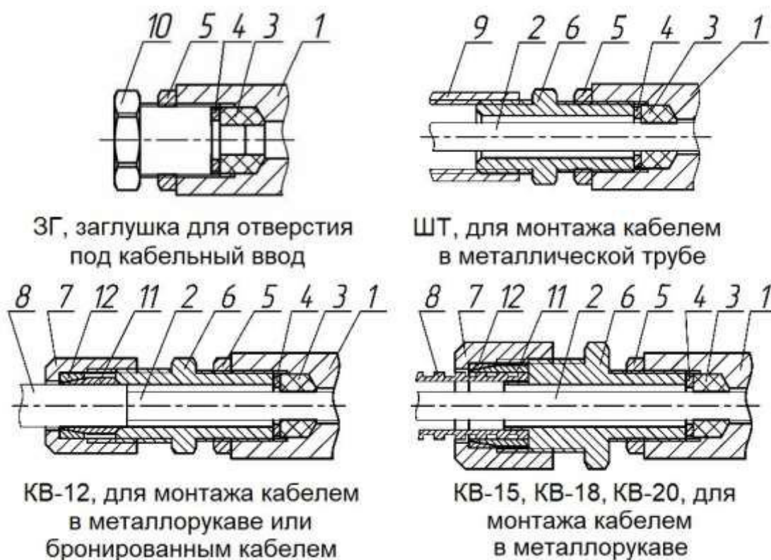
Рисунок 5 – Вводные устройства с одинарным уплотнением
