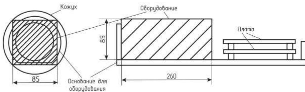
Рисунок 2 – Полезный объем термокожуха для установки видеооборудования Релион-ТКВ-ВО – 85х85х260 (габариты видеооборудования)
