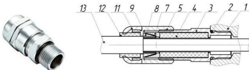
KB-BK-12 – монтаж бронированным кабелем
