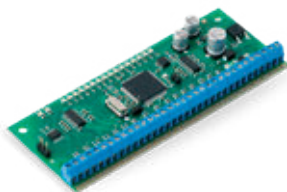
ЕРGM1 - модуль расширения проводных зон и ПГМ выходов
