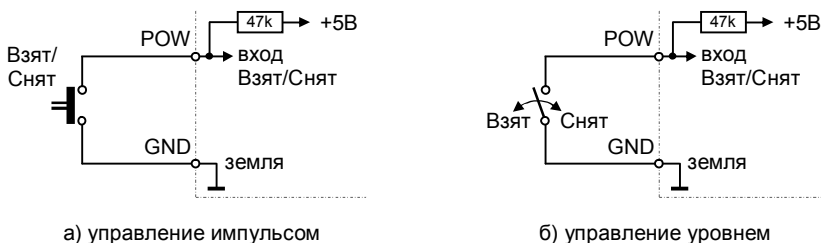
Рисунок 3 – Монтажная схема линии Взят/Снят
