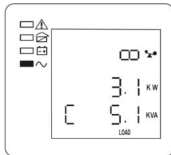
Рисунок 16 — ЖК-дисплей, Фаза С, величина нагрузки
