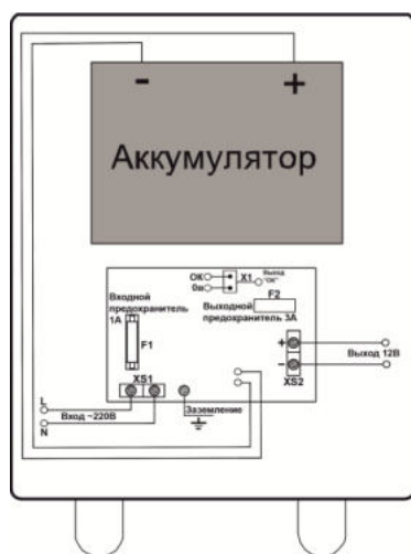
Схема подключения рис. 1
