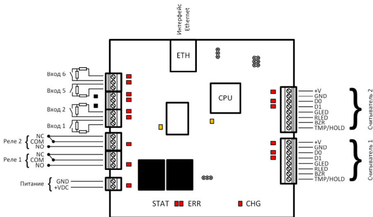
Назначение контактов контроллера ST-NC221
