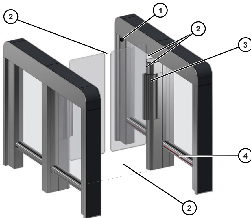
Рис. 2: Защитные устройства установки Argus 40
