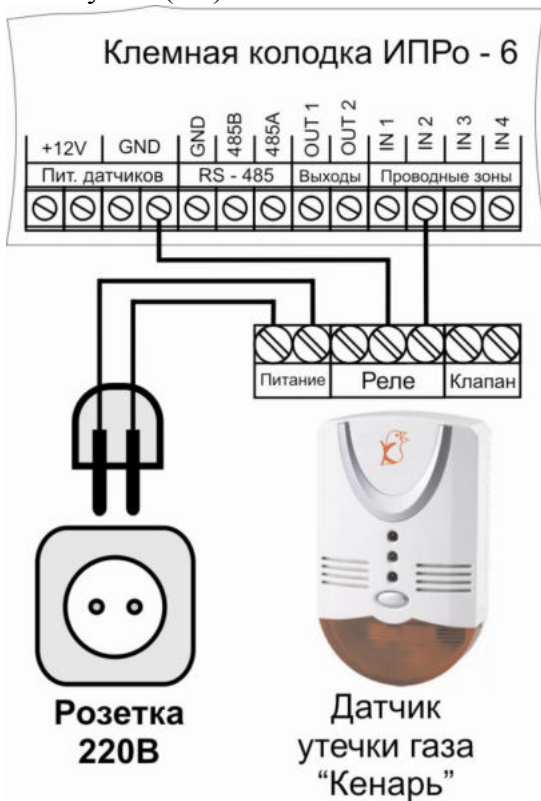
Подключение 1 датчика
