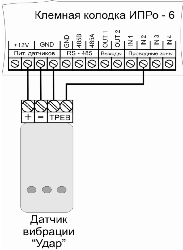
Подключение 1 датчика
