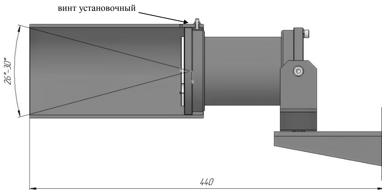
Рис. 2 – Установка бленды на извещатель, положение №1
