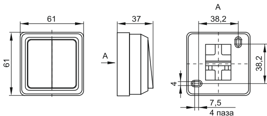
Рисунок 2. Габаритные размеры выключателей.
