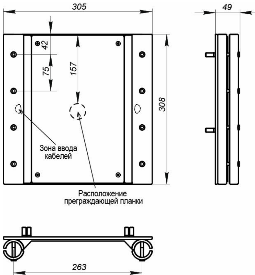
Рисунок 14. Кронштейн PERCo-MT10.1 в сборе, внешний вид и габаритные размеры
