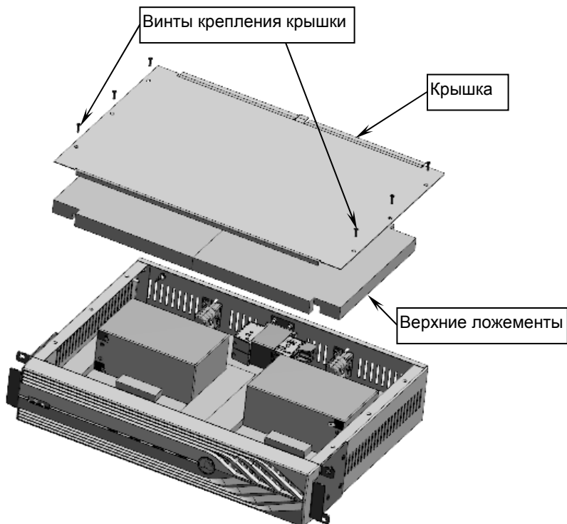
Рисунок 6 — Замена аккумуляторных батарей.
