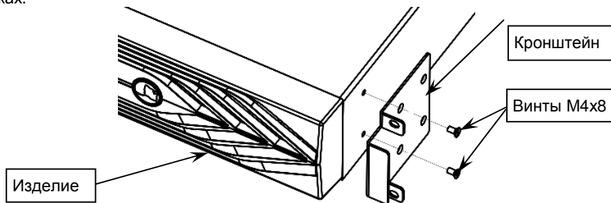
Рисунок 4 — Установка кронштейнов на корпус изделия
