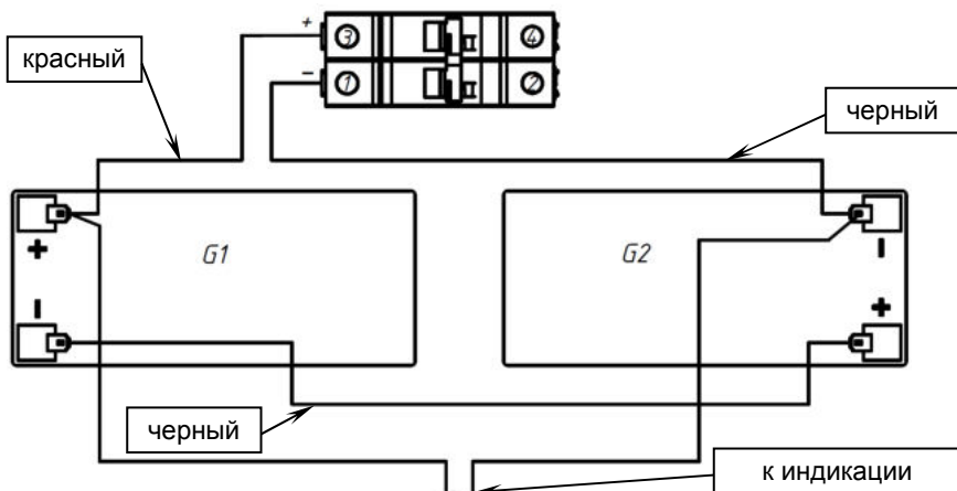
Рисунок 7 — Схема соединений аккумуляторных батарей
