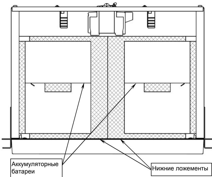
Рисунок 3 – Размещение аккумуляторных батарей в корпусе
