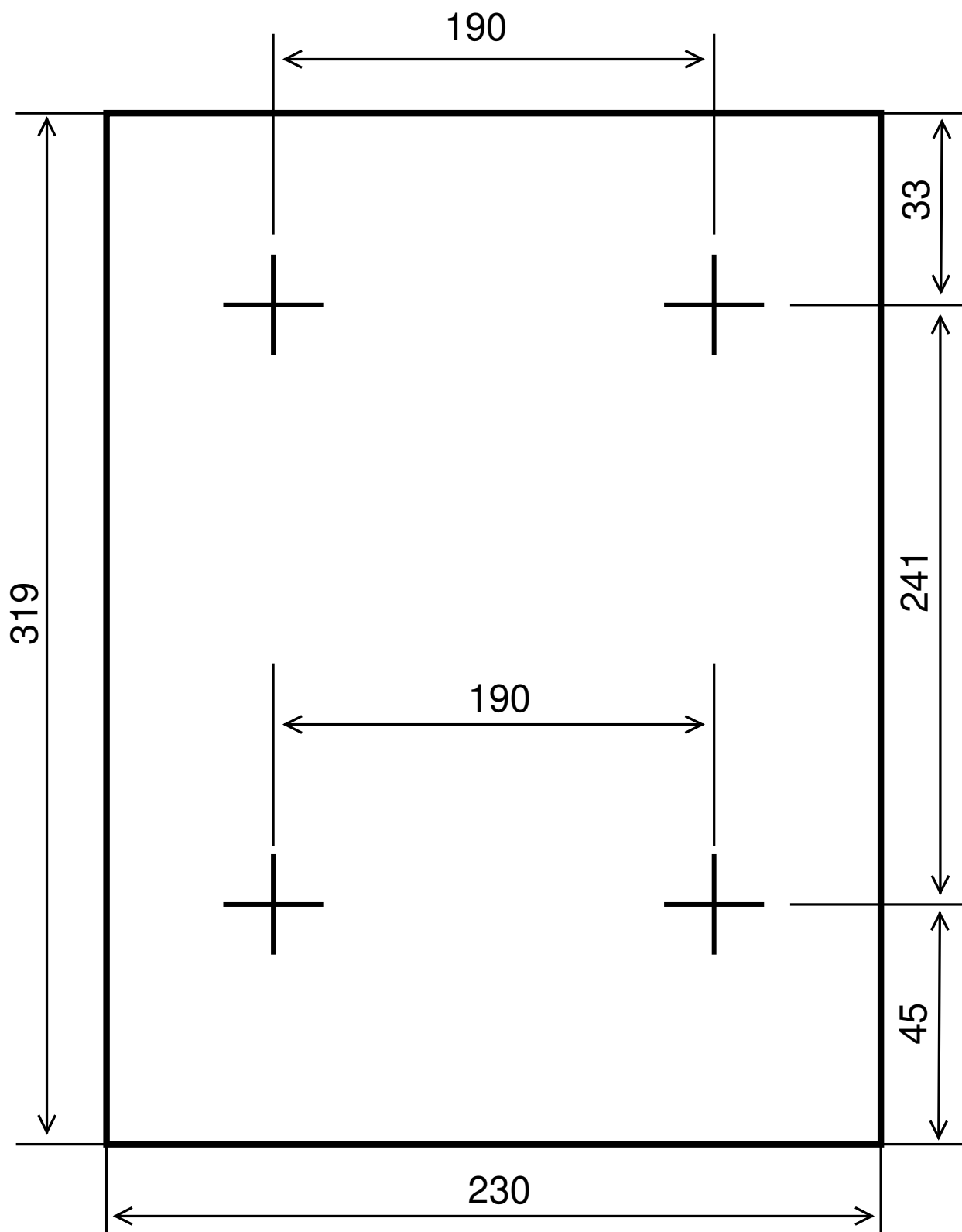
Габаритно-установочные размеры РИП
