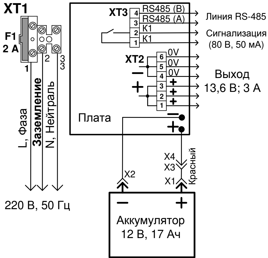
Схемы внешних подключений
