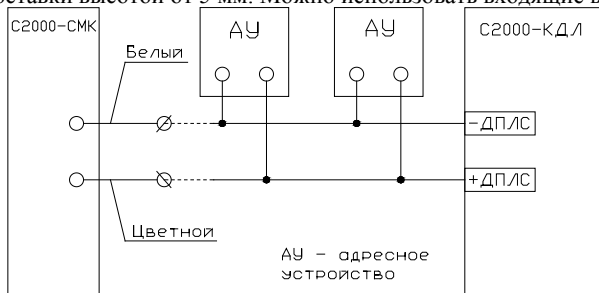
Рисунок 1 Схема соединений
