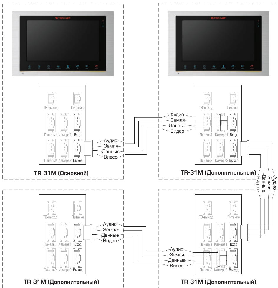
Схема 2. Подключение системы мониторов TR-31M
