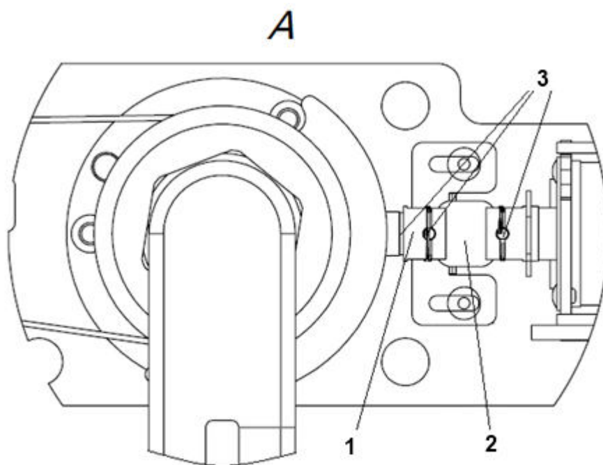
1 - фиксатор; 2 - серьга; 3 - 2-3 капли масла
