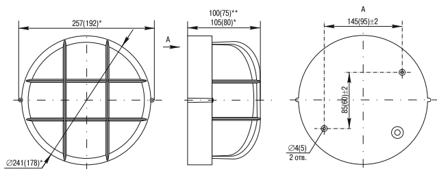
Рисунок 1 – Габаритные и установочные размеры светильников НПП 1102...1108
