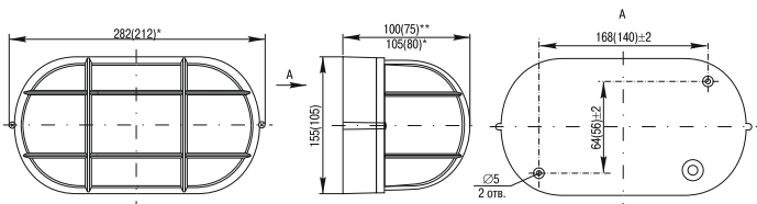
Рисунок 2 – Габаритные и установочные размеры светильников НПП 1202...1208
