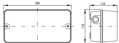
Рисунок 4 – Габаритные и установочные размеры светильника НПП 3006
