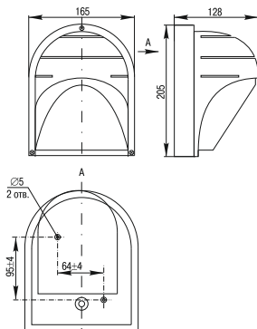
Рисунок 3 – Габаритные и установочные размеры светильника НПП 2501
