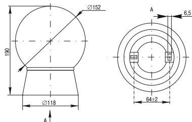
Рисунок 5 – Габаритные и установочные размеры светильника НПП 9101
