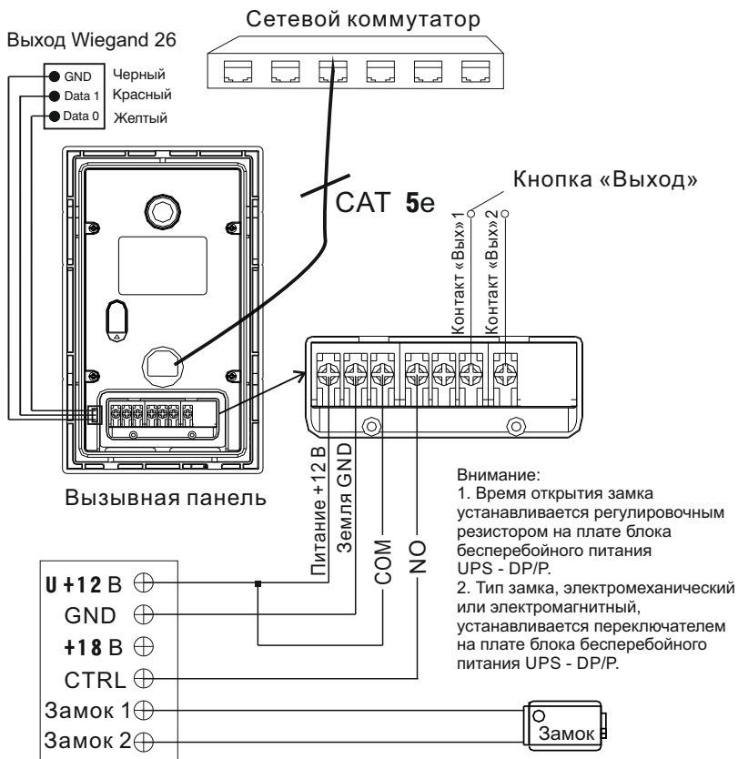
Блок Бесперебойного Питания (UPS-DP/P)
