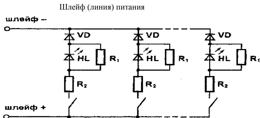
Рис. 4.. Эквивалентная схема при включении извещателя ИПР513-2 «АГАТ» P1 (P2) по варианту, аналогичному типовой схеме включения дымового или иного токопотребляющего пожарного извещателя в четырёхпроводный шлейф сигнализации, при этом:
